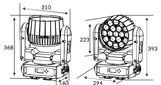
寸法図
