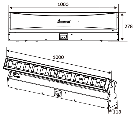
寸法図(mm)
