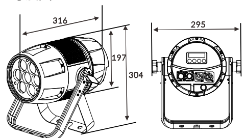
寸法図
