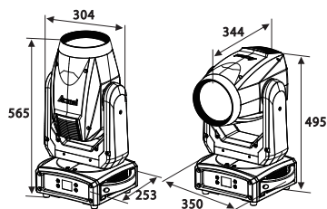
寸法図(mm)
