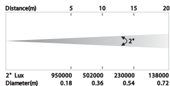
照度図
